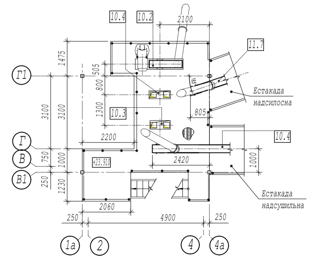
План майданчика на відм.+23.910
