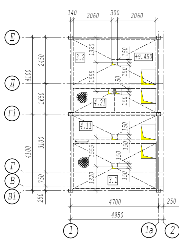
План майданчика на відм.+9.450
