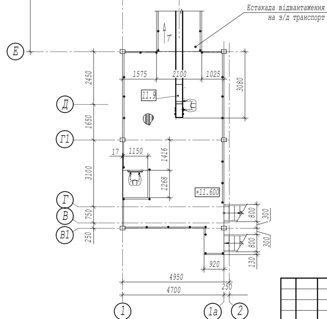
План майданчика на відм.+11.600
