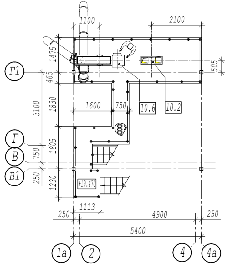
План майданчика на відм.+19.470
