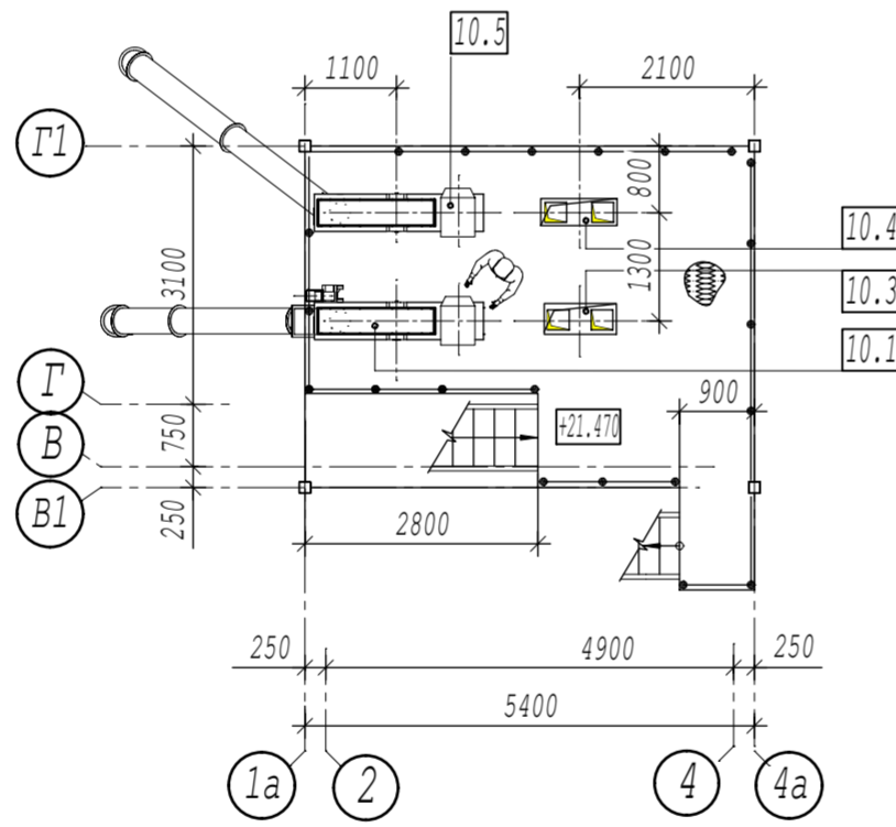
План майданчика на відм.+21.470
