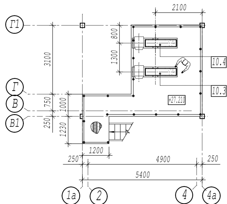
План майданчика на відм.+27.210
